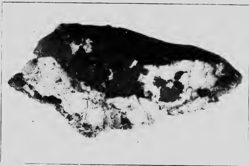
Partie d'une lentille de minéral, mines de tungstène de Moose River. — Ardoise noire, arsénio-pyrite gris foncé, quartz blanc clair. — Le blanc terne qui forme la partie supérieure du dessin est de la scheelite.
